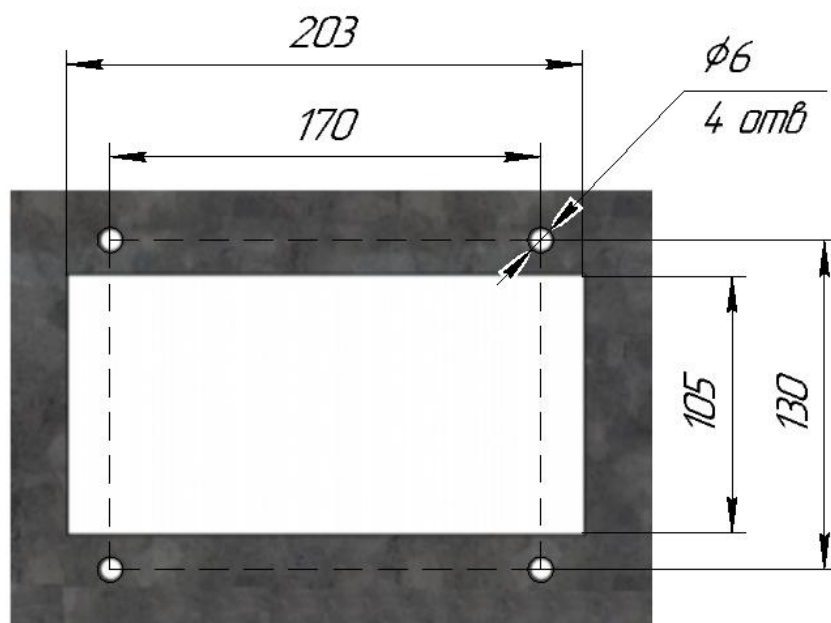
Рисунок 5. Размеры отверстия в стенке основания для установки пульта управления.
