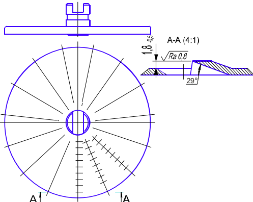
Рисунок 7 — Диск тёрочный
