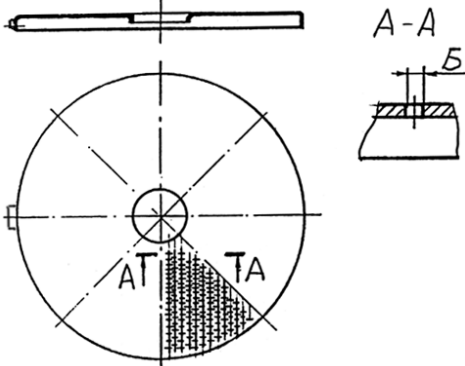
Рисунок 10 — Диск протирочный
