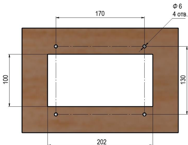
Рисунок 4. Размеры отверстия в стенке основания для установки пульта управления.
