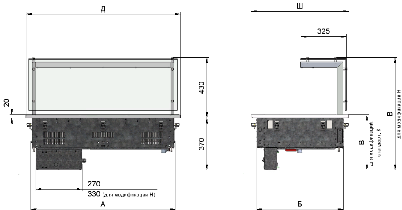
Рисунок 3. Основные габаритные размеры оборудования.
