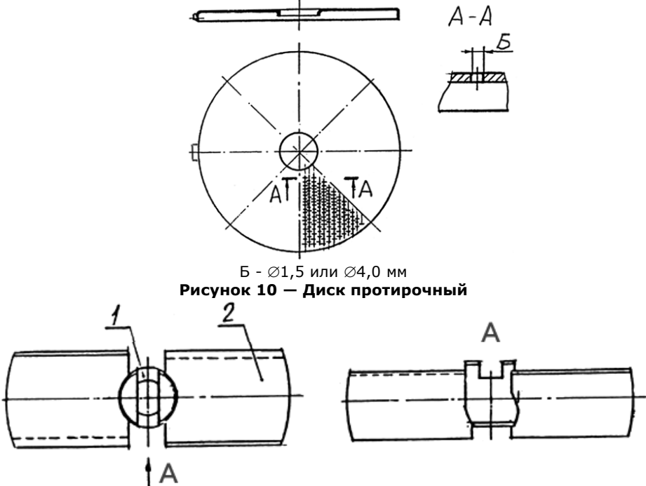
1 - втулка; 2 - лопасть Рисунок 11 — Ротор лопастной
